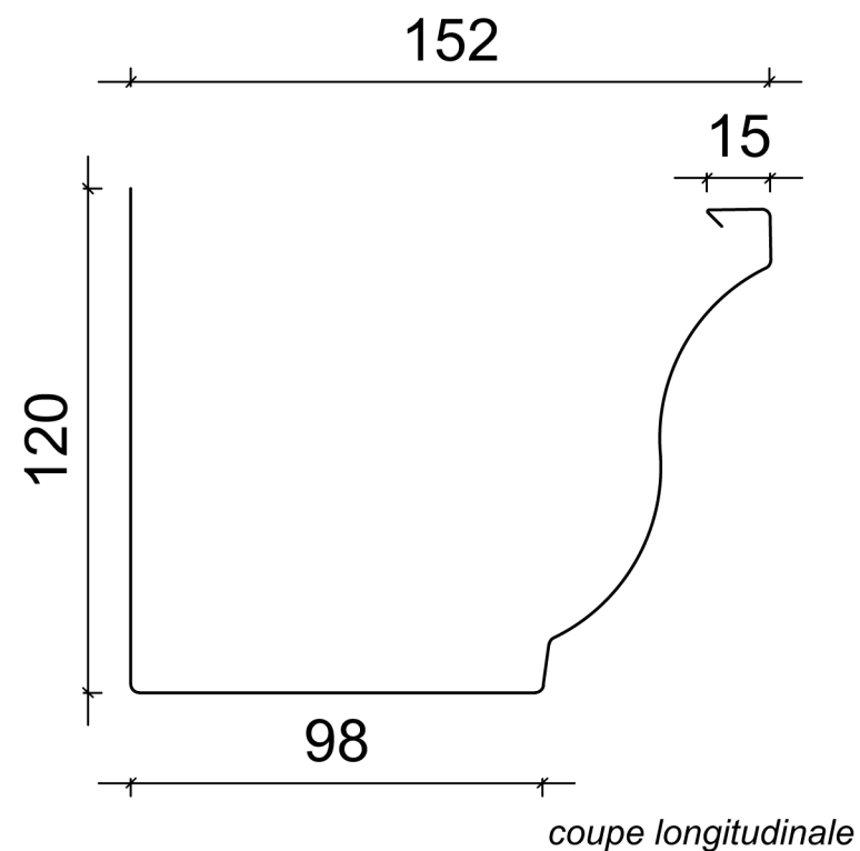
Profil G380
